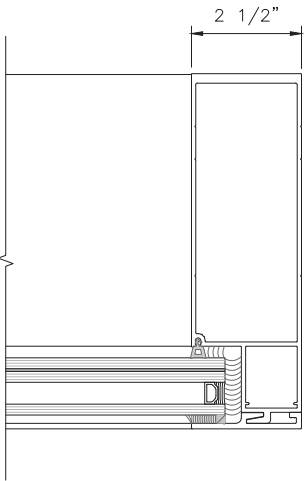
JAMB (J1)
